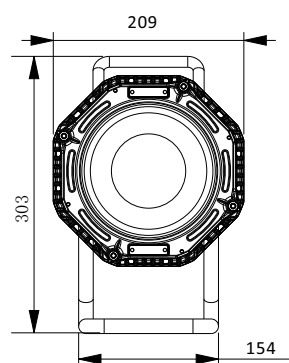
Art.-Nr.: 321174 FlutLED Ex 10W mit Bodengestell
