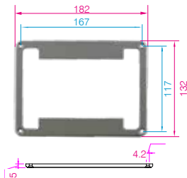
Manschette für Doppeldecken und Doppelböden
