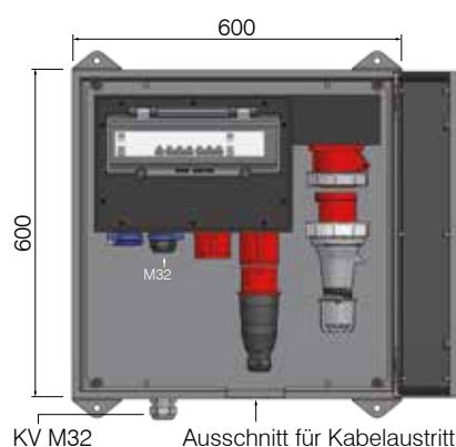
KV M32 Ausschnitt für Kabelaustritt
