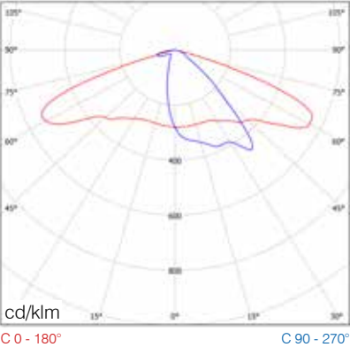
Lichtverteilung 65W – 10325lm
