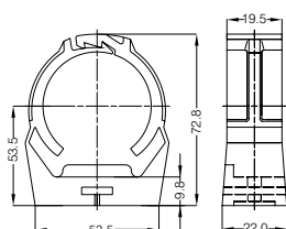
Wandhalterung SL POWER, Art.-Nr. 282492
