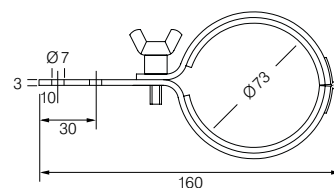
Wandhalterung SL70 Typ 3, Art.-Nr. 840085
