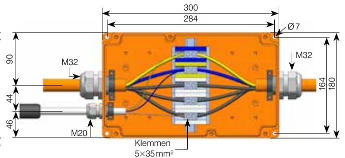
Baureihe 3018 – 300×180×100 mm / 5×35 mm 2 Art.-Nr.: 189886
