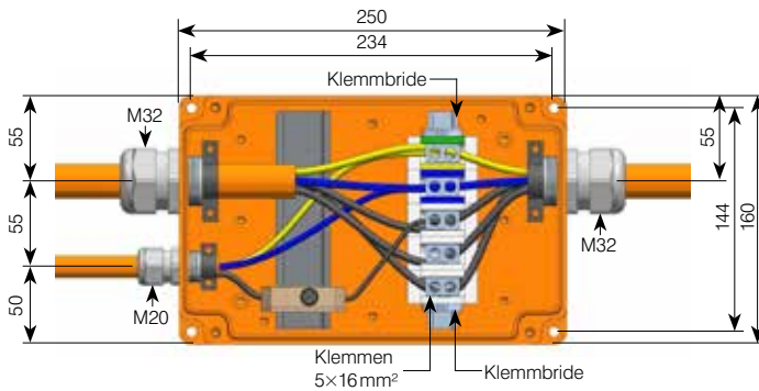
Baureihe 2516 – 250×160×100 mm / 5×16 mm 2 Art.-Nr.: 205665
