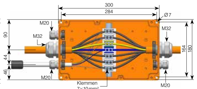
Baureihe 3018 – 300×180×100 mm / 7×10 mm 2 Art.-Nr.: 189887
