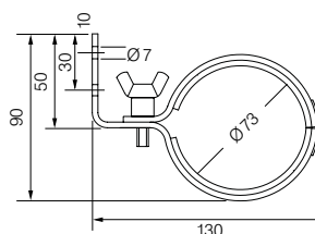
Wandhalterung SL70 Typ 1, Art.-Nr. 840083
