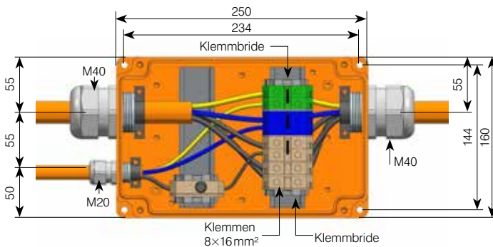
Baureihe 2516 – 250×160×100 mm / 8×16 mm 2 Art.-Nr.: 205666
