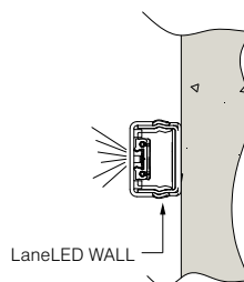
Schnitt A-A/C-C:
